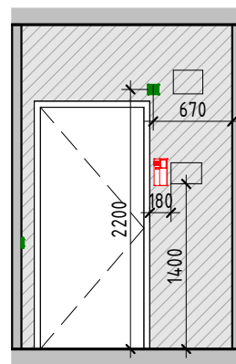
прихожая 3
