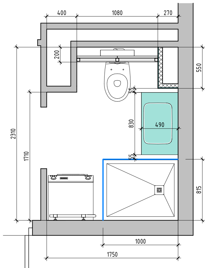
Чертеж ванны
