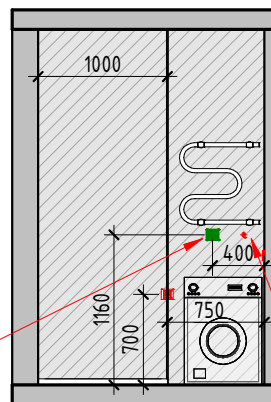
санузел 3
