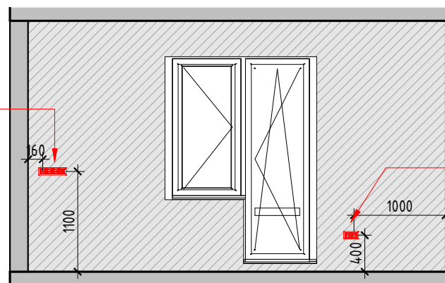
Балкон
